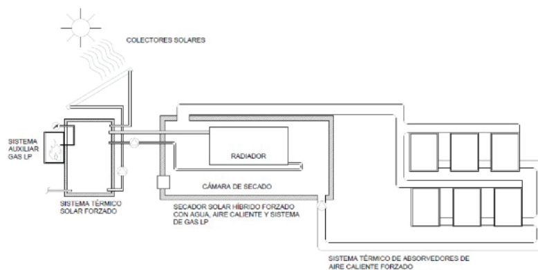
Figura 1. Secador solar híbrido forzado con gas LP. (Fuente. Uso de Energía solar en Actividades Agropecuarias de la Región Huetar Norte, pag 174) [10].
