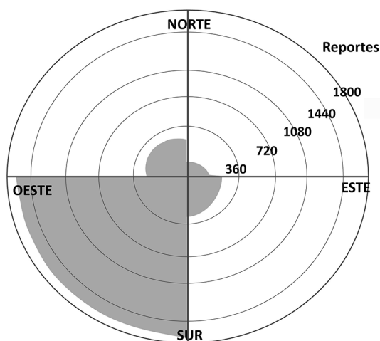
Fig. 7: Distribución de reportes por cada ceniza según dirección de los vientos, periodo 2010 – 2017.
