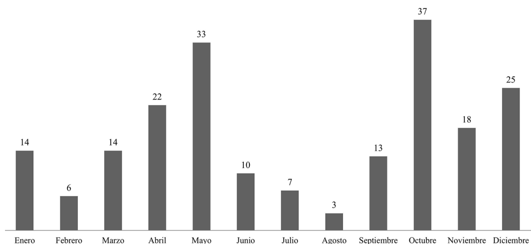
Fig. 6: Cantidad de erupciones reportadas por mes por caída de ceniza, periodo 2010-2017.
