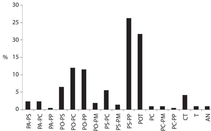
Fig. 2. Porcentajes de afinidad ictiogeográfica (PA: Provincia Aleutiana, PO: Provincia Oregoniana, PS: Provincia de San Diego, PC: Provincia de Cortés, PM: Provincia Mexicana, PP: Provincia Panámica, POT: Pacífico Oriental Tropical, CT: Especies Circumtropicales, T: Especies Transpacíficas, AN: Especies Anfiamericanas).
