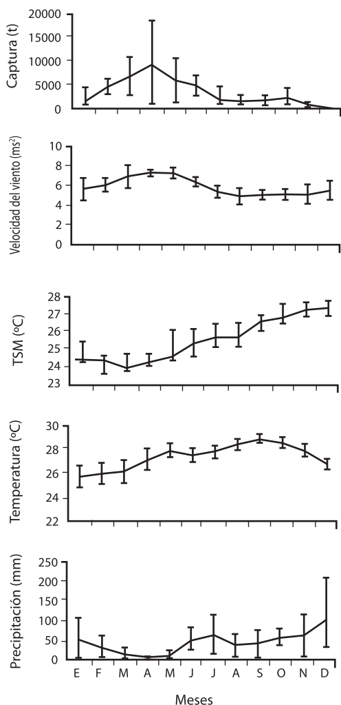
Fig. 2. Variación estacional de la captura de Sardinella aurita , velocidad del viento, temperatura superficial del mar, temperatura del aire y precipitación en El Morro, durante 1996-2000.
