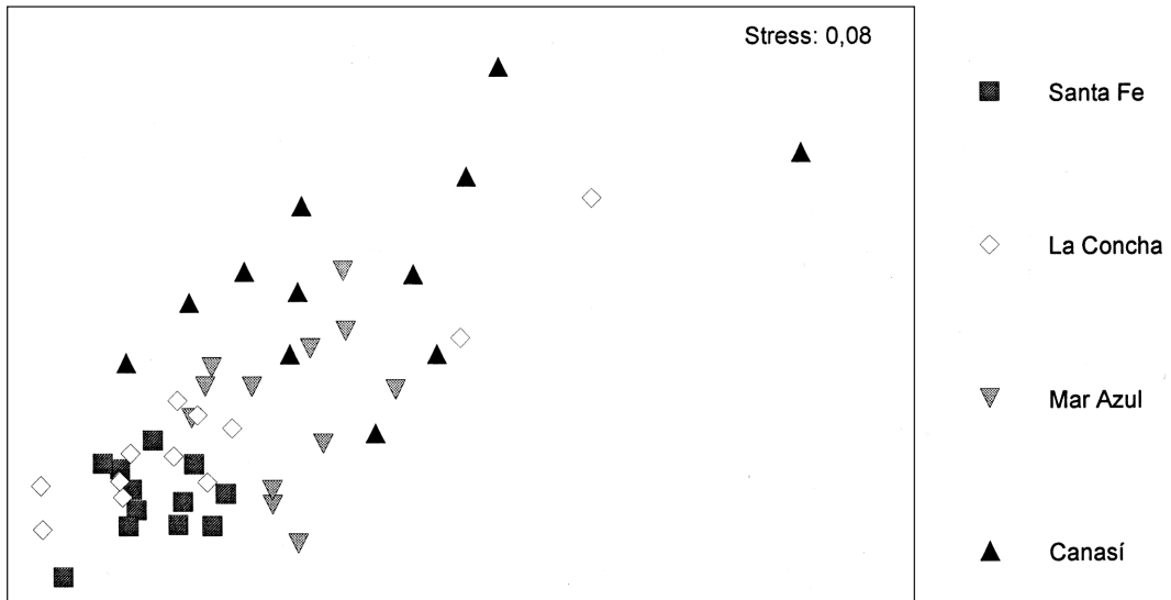
Fig. 4. Agrupación mensual de las estaciones.
