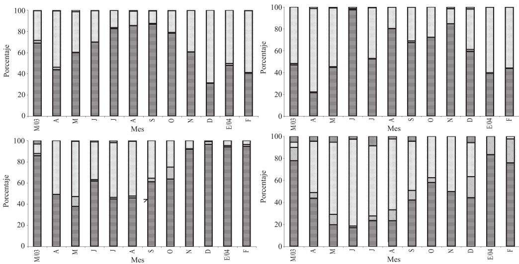
Fig. 2. Porcentaje de la densidad de grupos de la meiofauna anual y mensual. Santa fe (A), La Concha (B), Mar Azul (C) y Canasí (D).
