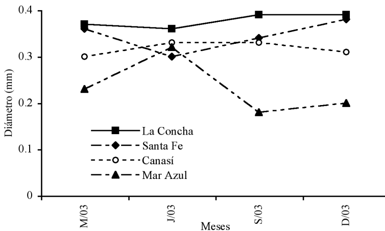
Fig. 1. Diámetro medio de las partículas de arena.
