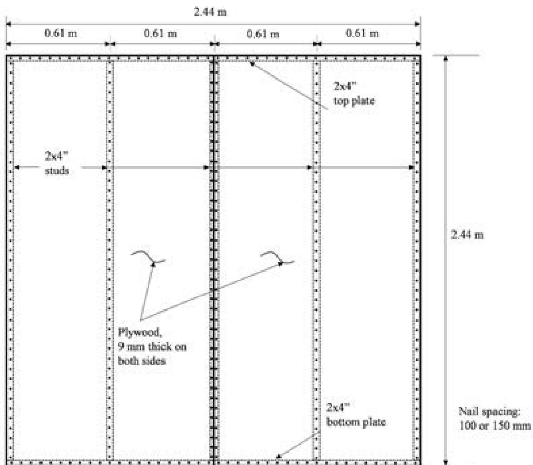
Fig. 1. Test specimen.
