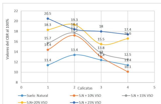
Figura 8. Resultados del ensayo de CBR al 100% según porcentajes de vinaza de Saccharum officinarum adicionados a las muestras de suelo
