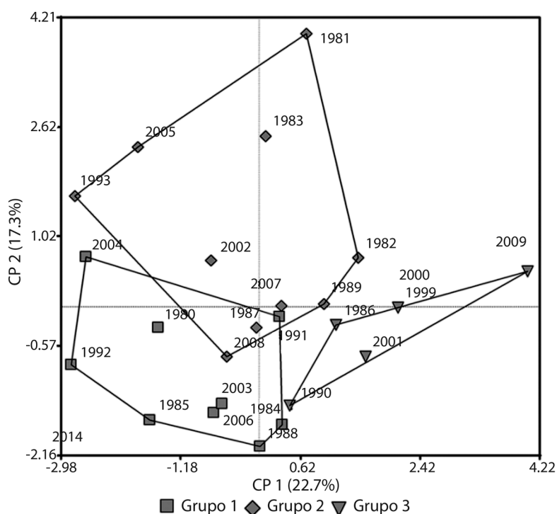
Fig. 3. Combinación del análisis de coordenadas principales y análisis de conglomerados para la serie temporal 1980-2014 del SPI en Banco de San Pedro estado Guárico.
