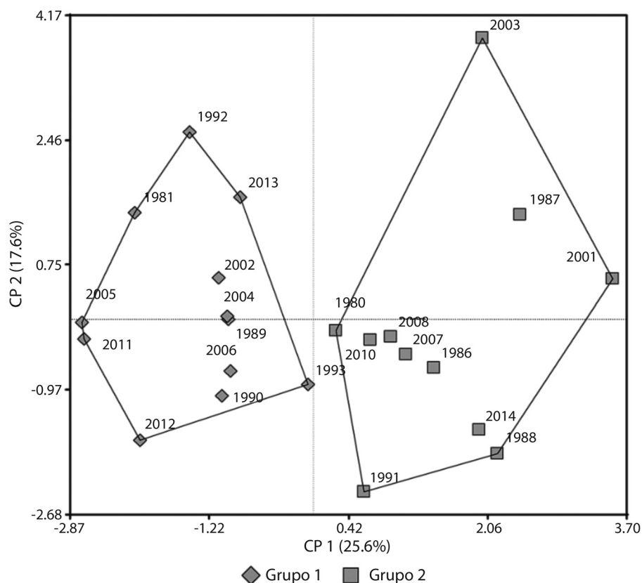
Fig. 4. Combinación del análisis de coordenadas principales y análisis de conglomerados para la serie temporal 1980-2014 en Tapipa-Padrón estado Miranda.
