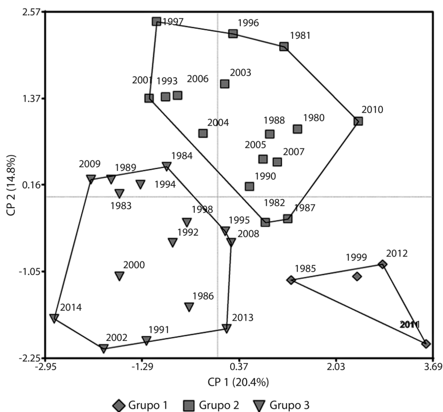
Fig. 2. Combinación del análisis de coordenadas principales y análisis de conglomerados para la serie temporal 1980-2014 del SPI en El Tígr estado Anzoátegui.
