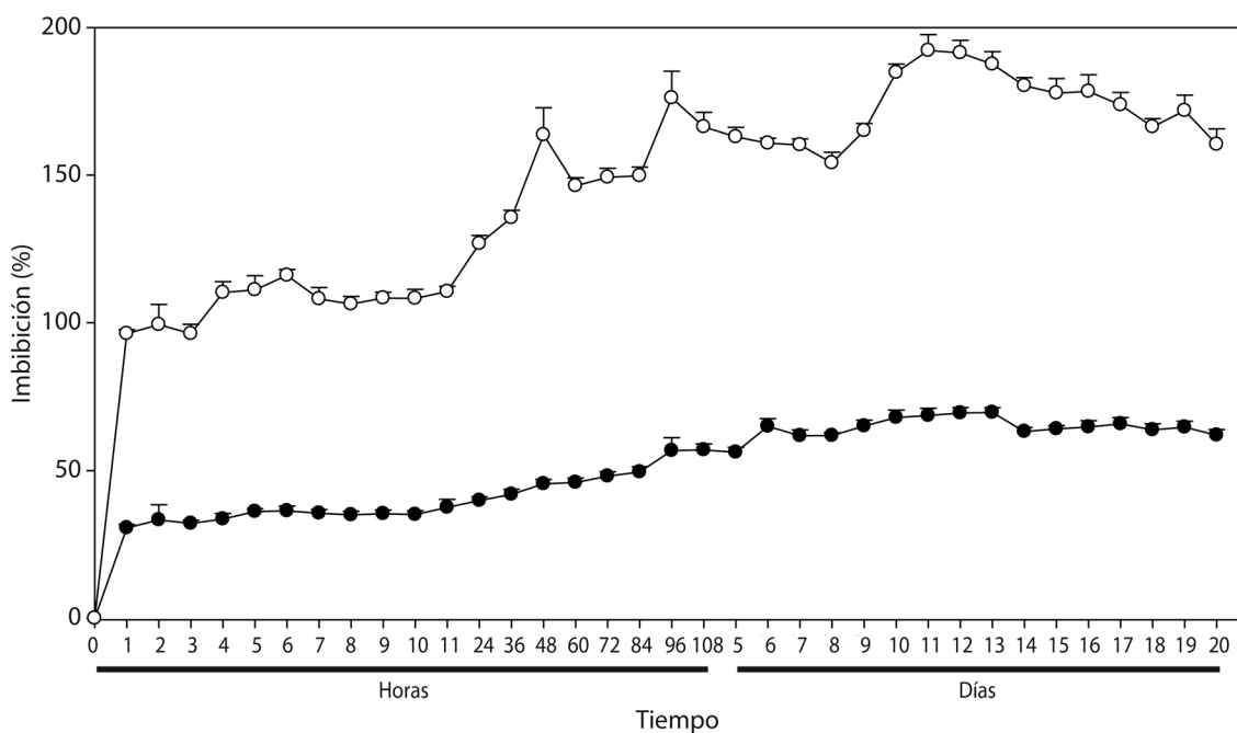
Fig. 2. Dinámica de imbibición, en lotes de 100 endocarpios sin escarificar de (—○—) Malpighia mexicana A. Juss. y (—●—) Byrsonima crassifolia (L.) H. B. K.
