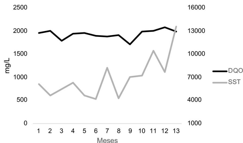
Figura 1. Variación mensual de la demanda química de oxígeno (DQO) y los sólidos suspendidos totales (SST) en las aguas de lavado. Universidad de Costa Rica, Turrialba, Costa Rica. Mayo 2022-mayo 2023.
