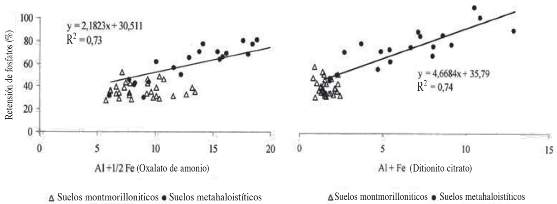
Fig. 5. Relación entre % de retención de fosfatos y la concentración de Al y Fe extraídos con Oxalato de amonio y ditionito citrato en suelos de las familias montmorillonítica y metahalostífica.
