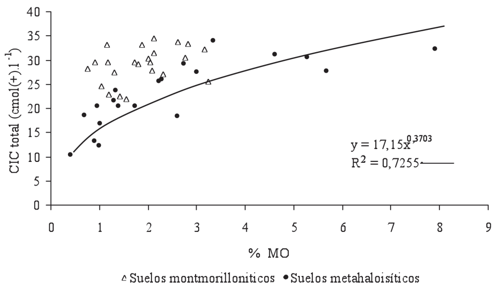
Fig. 2. Relación entre CIC y el % de MO en suelos de las familias montmorillonítica y metahalosíctica.
