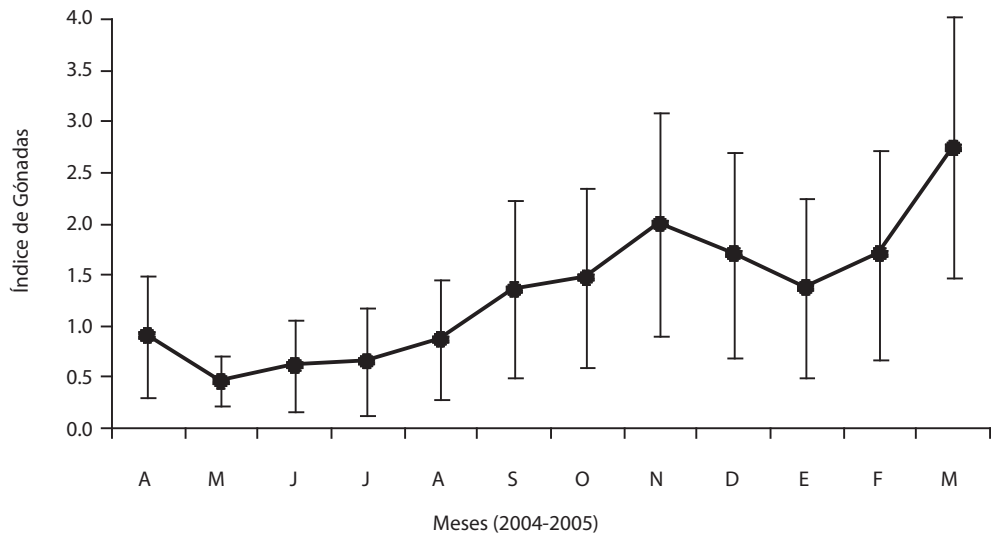
Fig. 3 Variación mensual de índice de gónadas de Sardinella aurita del sureste de la Isla de Margarita de abril 2004 a abril 2005.
