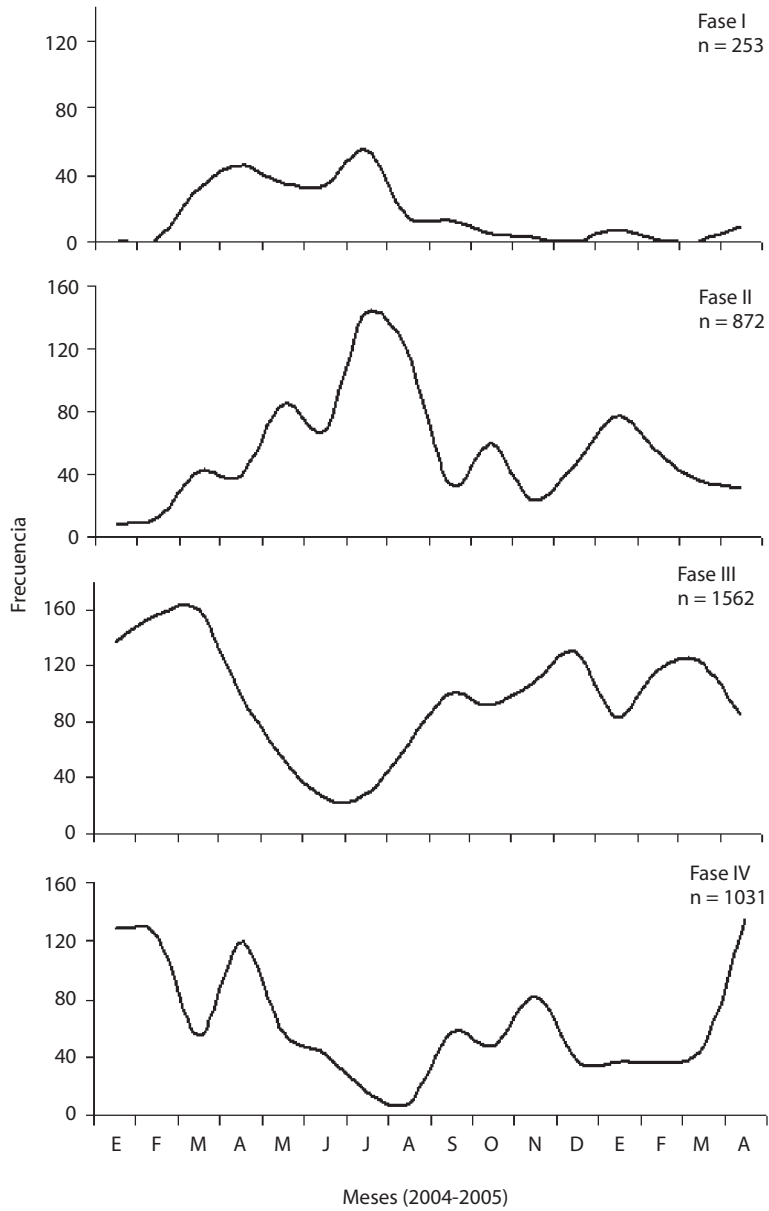
Fig. 2 Variación mensual de la frecuencia absoluta de las fases de madurez sexual de Sardinella aurita del sureste de la Isla de Margarita de enero 2004 a abril 2005.
