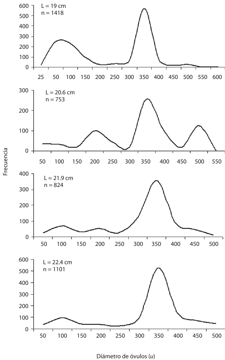
Fig. 5 Distribución de frecuencia del diámetro de óvulos en ovarios de hembras maduras de diferentes longitudes de Sardinella aurita del sureste de la Isla de Margarita
