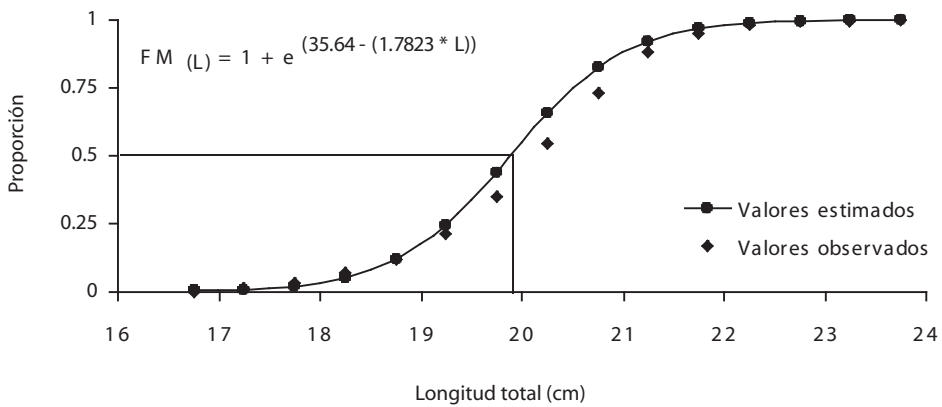
Fig. 4 Talla media de madurez sexual de la población ( L_{50} ) de Sardinella aurita del sureste de la Isla de Margarita.
