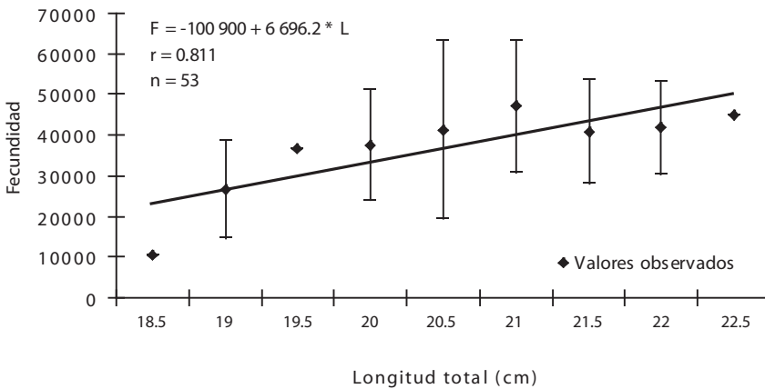
Fig. 6 Relación entre la fecundidad absoluta y la longitud total de Sardinella aurita del sureste de la Isla de Margarita.
