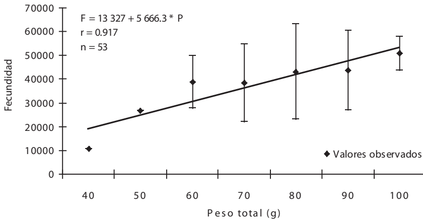
Fig. 7 Relación entre la fecundidad absoluta y el peso total de Sardinella aurita del sureste de la Isla de Margarita.
