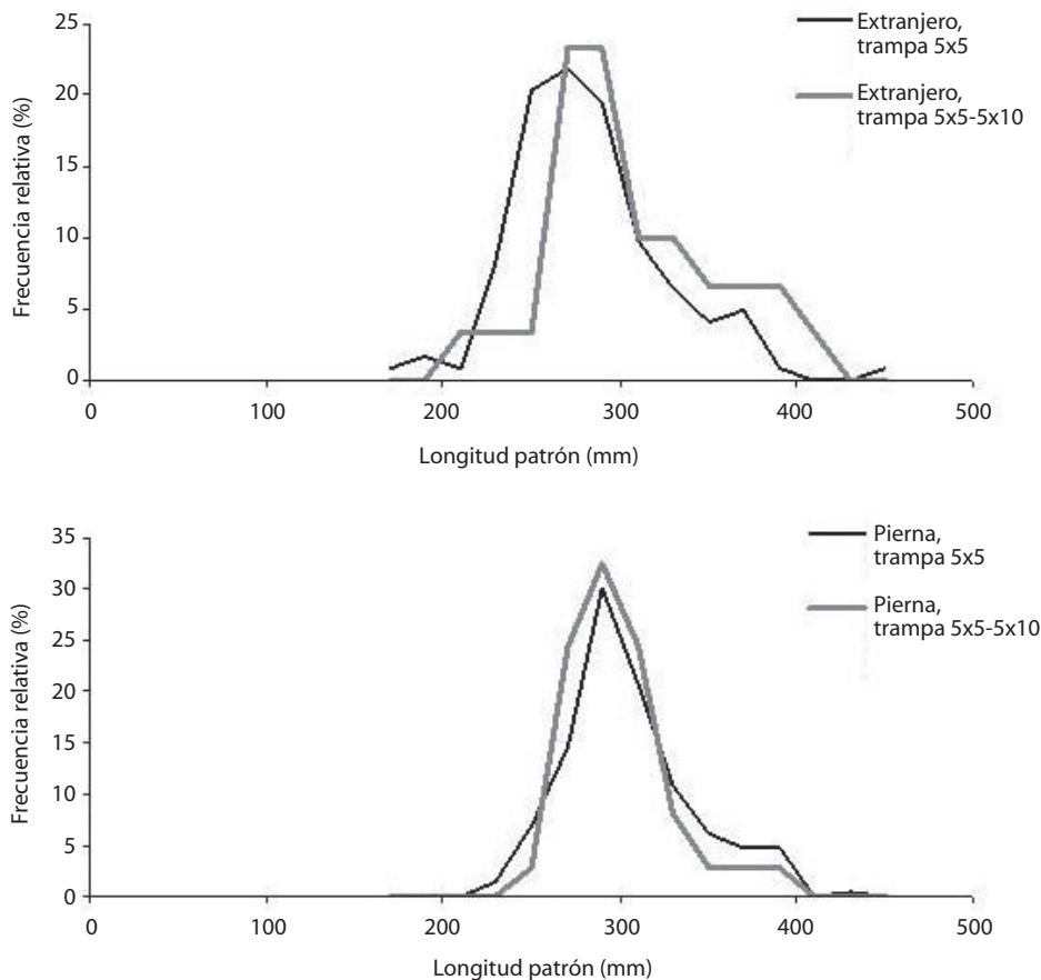
Fig. 5. Distribución de frecuencias de tallas del extranjero ( Paralabrax auroguttatus ) y pierna ( Caulolatilus princeps ) capturados en trampas en Guaymas, Sonora, México.
