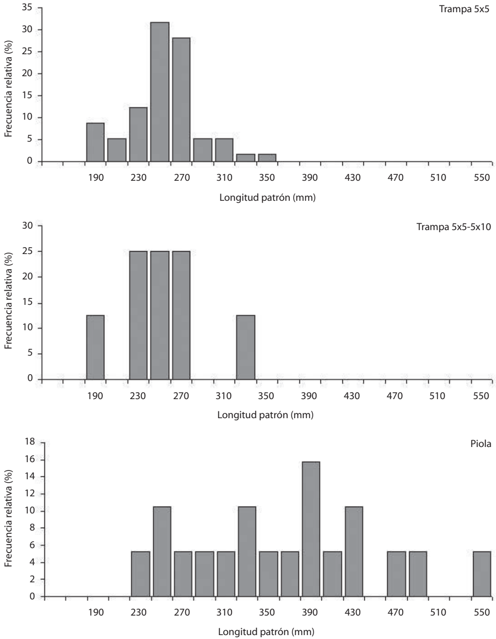
Fig. 3. Distribución de frecuencias de tallas de peces en trampas y piola de mano con anzuelo en Yavaros, Sonora, México.
