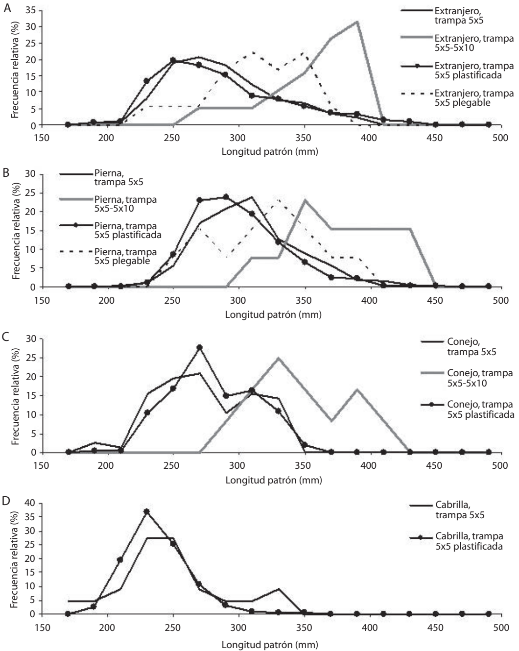
Fig. 6. Distribución de frecuencias de tallas de extranjero ( Paralabrax auroguttatus ), pierna ( Caulolatilus princeps ), conejo ( C. affinis ) y cabrilla ( P. maculatofaciatus ) capturados en trampas en Kino, Sonora, México.
