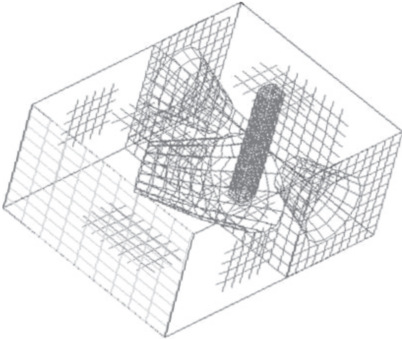
Fig. 1. Trampa de 5x5 cm, con panel trasero de malla de 5x10 cm, para la pesca de peces marinos.
