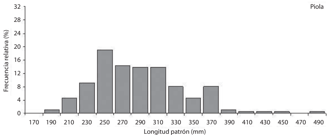
Fig. 2. Distribución de frecuencias de tallas de peces capturados en trampas y piola de mano con anzuelo en Guaymas, Sonora, México.
