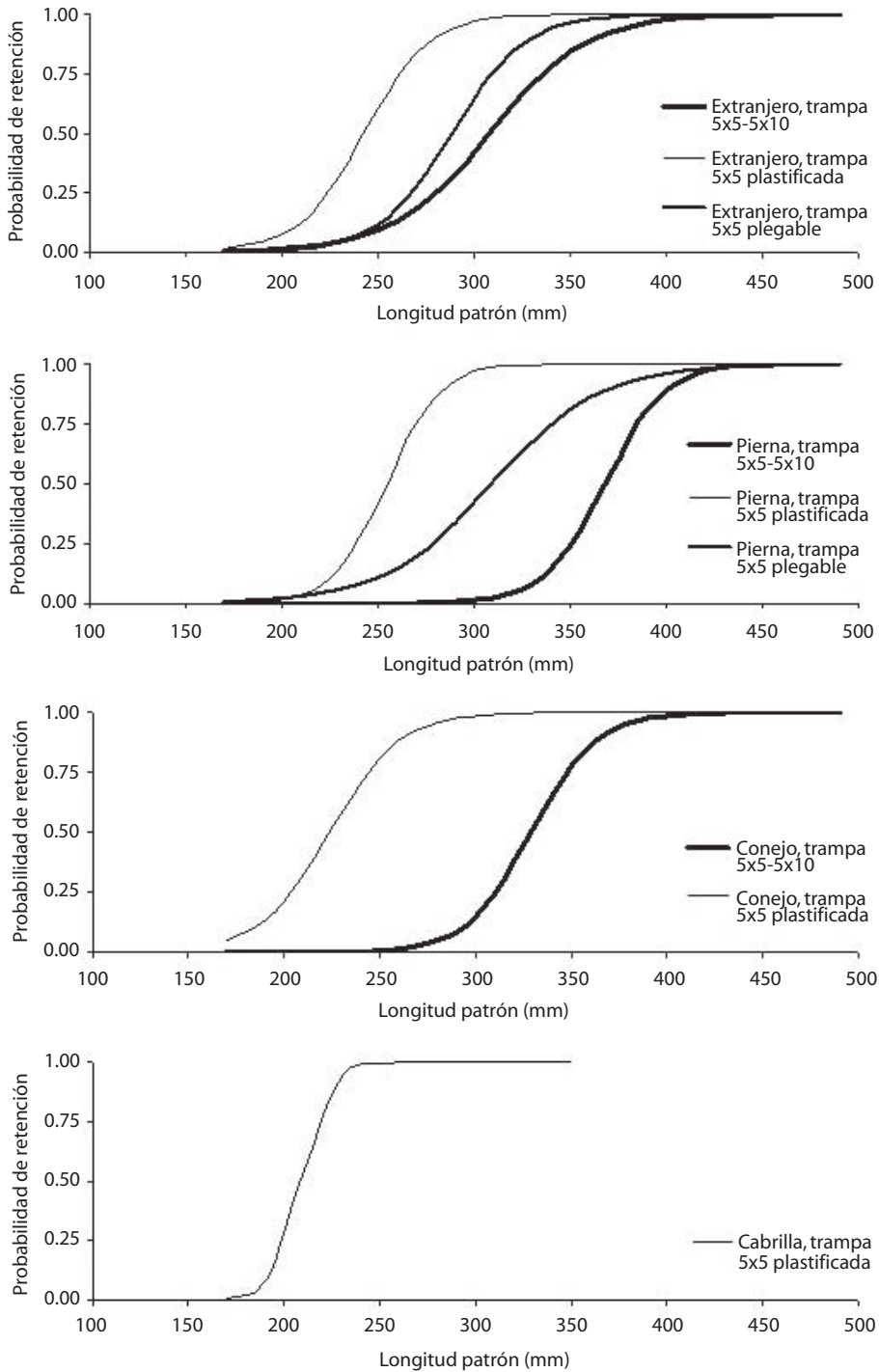
Fig. 7. Curvas de selectividad para cada tipo de trampa por especie en Kino, Sonora, México.
