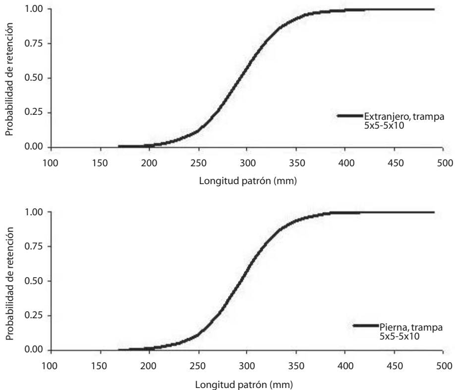
Fig. 8. Curvas de selectividad para cada tipo de trampa por especie en Guaymas, Sonora, México.
