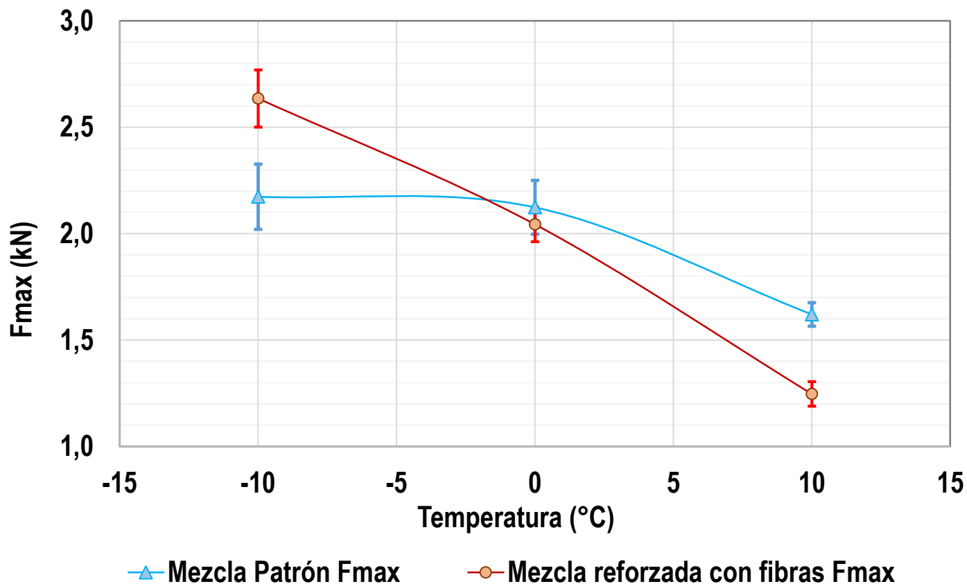
Figura 5 Resistencia a la fisuración vs temperatura
