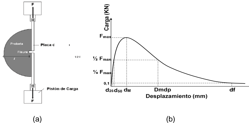
Figura 2 Ensayo FENIX. (a) Montaje ensayo Fénix, (b) Gráfica carga- desplazamiento. Fuente: (Valdés et al., 2009)
