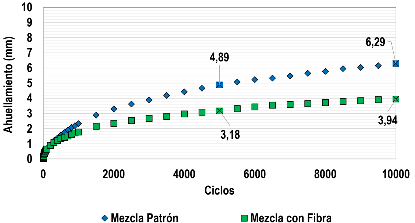
Figura 10 Curva de ahuellamiento de la mezcla patrón y mezcla reforzada con fibras sintéticas.
